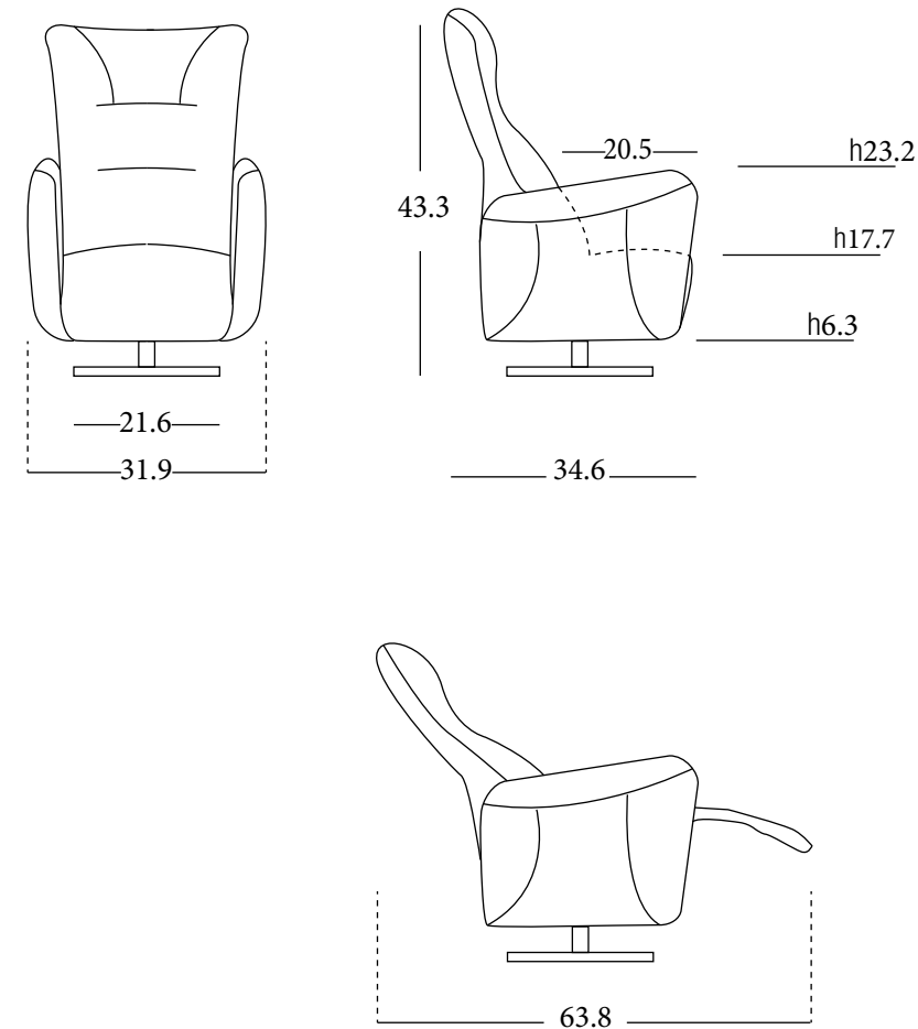
cod. 1170 POLTRONCINA GIREVOLE 2 MOT.
